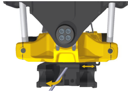
Afbeelding18. Draai de snelwissel naar links.
