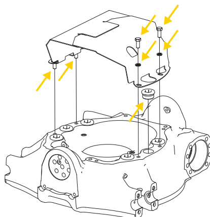
Afbeelding15. Demonstreer de beschermkap.
